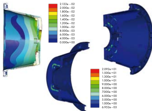
Stress berekening van een lantaarnstuk Strength calculation of a bellhousing
