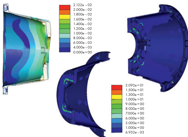
Расчет на прочность стойки насосов Strength calculation of a bellhousing
