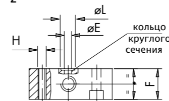
► AHM 1/2 - S ... боковое подключение
