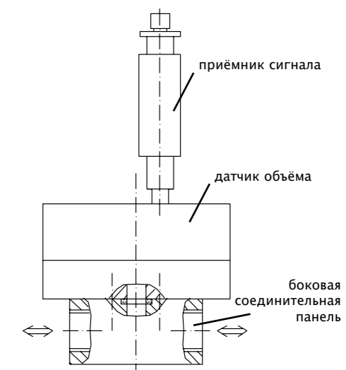
► Положение соединительных проводов
